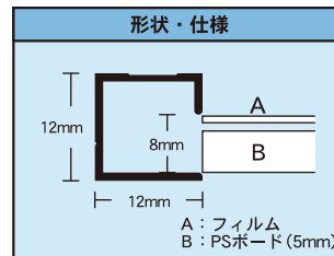
分解図
